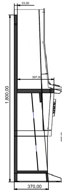
SECCIÓN A - A'
