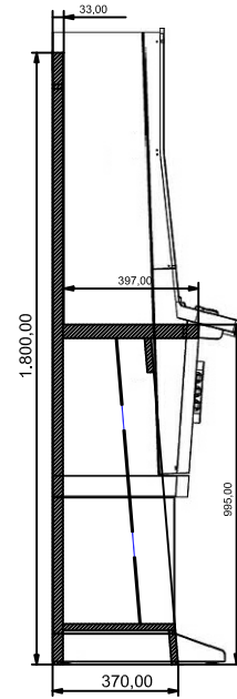
SECCIÓN A - A'
